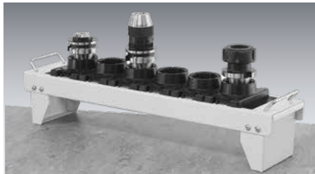
Dimensions LxPxH (mm) 590 x 125 x 110
